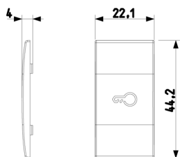
Dessin dimensions hors-tout
