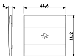
Dessin dimensions hors-tout
