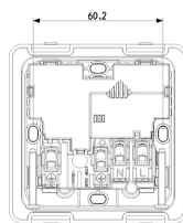
Vue arrière
