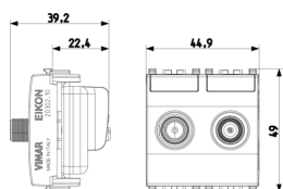
Dessin dimensions hors-tout
