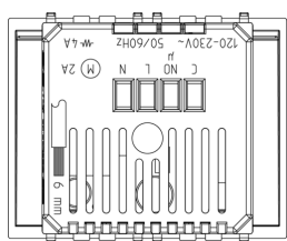
Vue arrière
