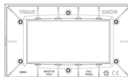
Vue arrière
