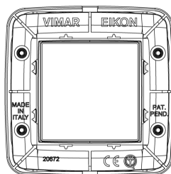
Vue arrière
