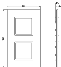
Dessin dimensions hors-tout
