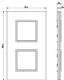
Dessin dimensions hors-tout
