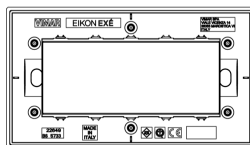
Vue arrière
