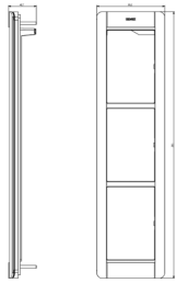
Dessin dimensions hors-tout
