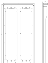
Dessin dimensions hors-tout
