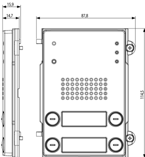
Dessin dimensions hors-tout
