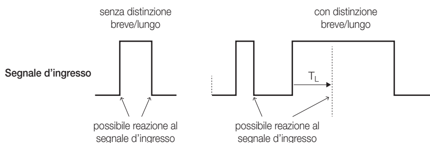
Fig. 1: distinzione tra azionamento breve/lungo della funzione "Commutazione"
