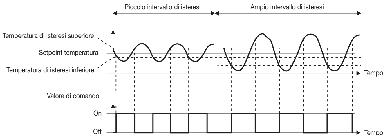
Figura 33 - Effetti dell'isteresi sul controllo (riscaldamento) in modalità di controllo a 2 punti
