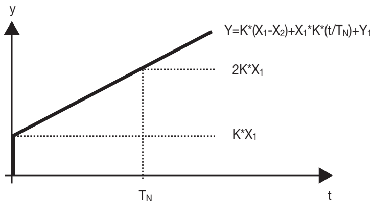
Figura 34 - Valore controllo per il PI
