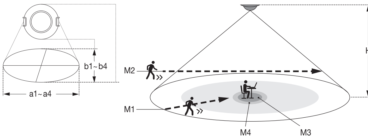
Figura 1 - Diagramma di installazione per 01527.2
