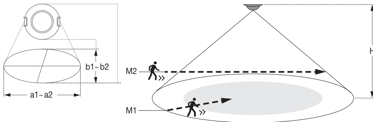
Figura 2 - Diagramma di installazione per 01529.2
