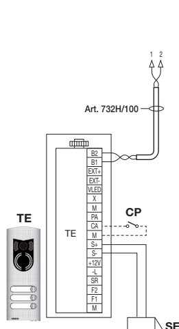
Figura 5 - Cerradura eléctrica de 12 Vcc y 200mA máx.
