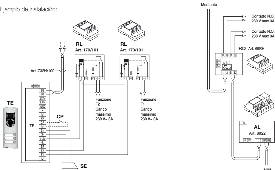
Figura 7 - Encendido de la luz de la escalera con FUNCIÓN F1/F2
