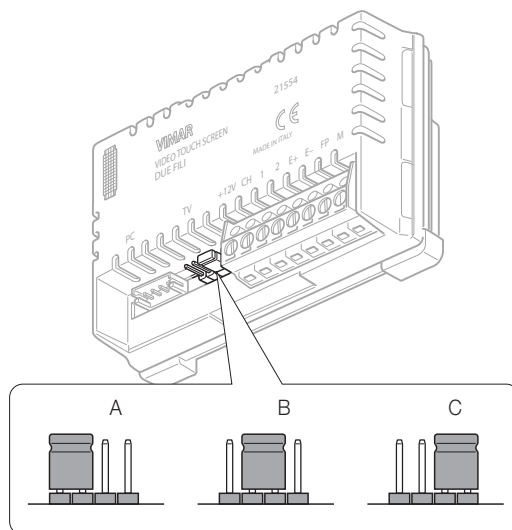
Figure 3 - Selector de terminación de la línea "TV"
