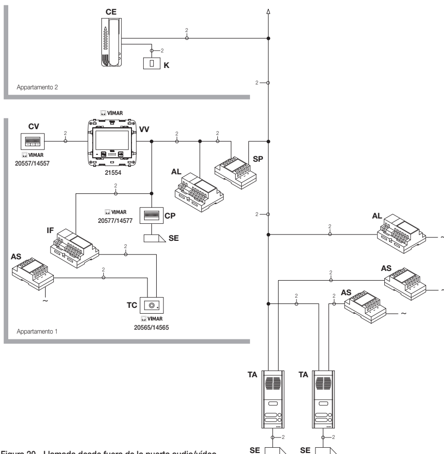
Figura 20 - Llamada desde fuera de la puerta audio/video
