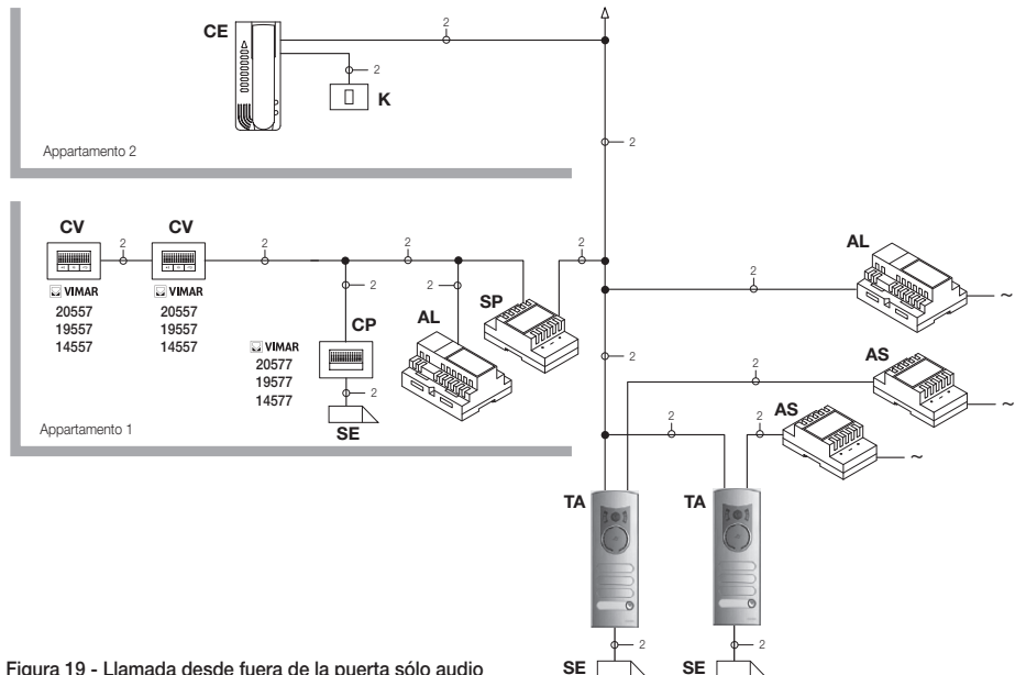
Figura 19 - Llamada desde fuera de la puerta sólo audio
