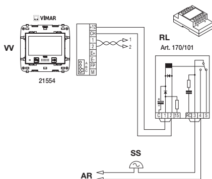
Figura 12 - Instalación de un timbre externo con relé
