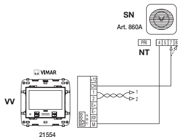
Figura 13 - Instalación de un timbre externo Elvox
