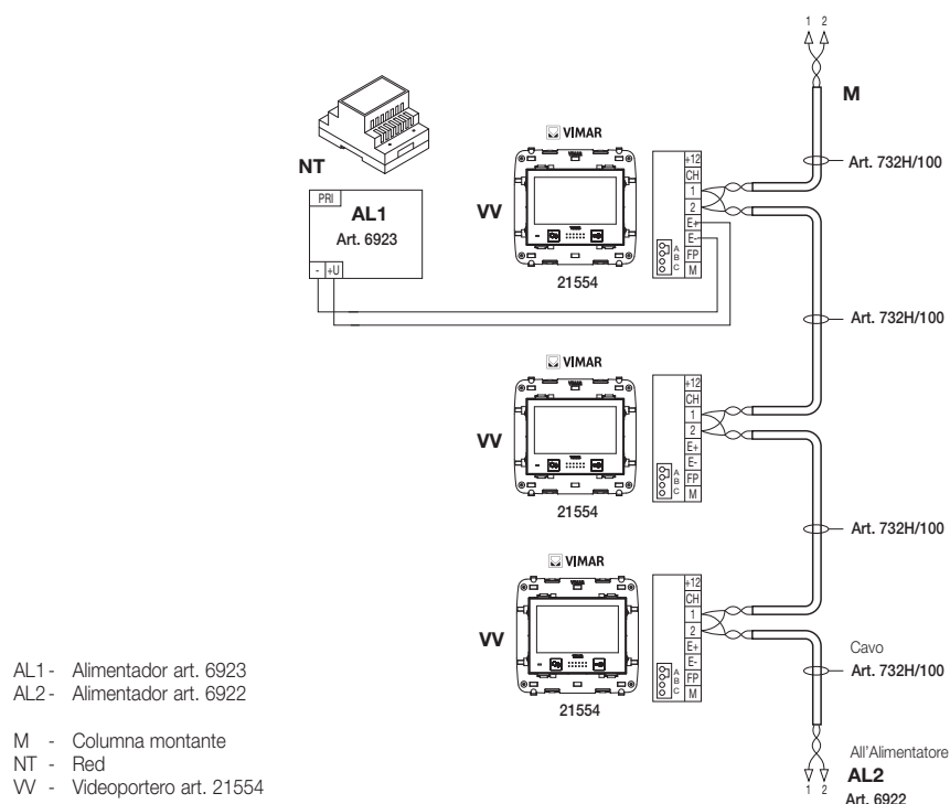
Figura 14 - Monitores con llamada de vídeo simultánea
