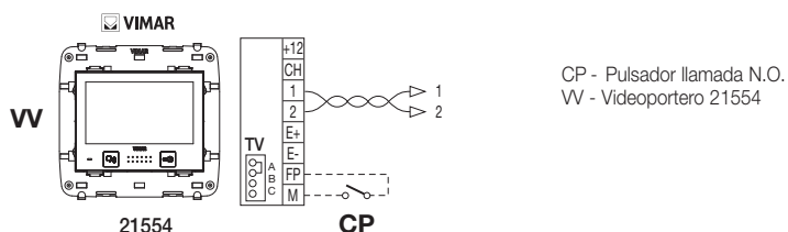
Figura 9 - Llamada desde timbre
