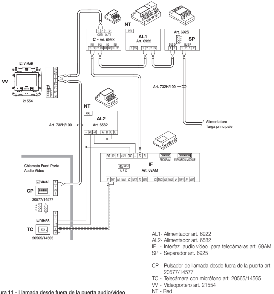
Figura 11 - Llamada desde fuera de la puerta audio/vídeo
