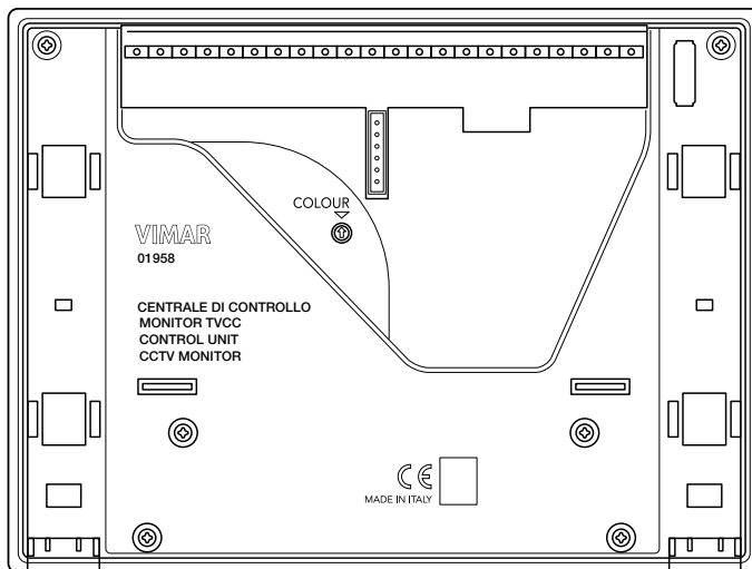
Figura 4 - Vista posteriore della centrale con monitor TVCC.
