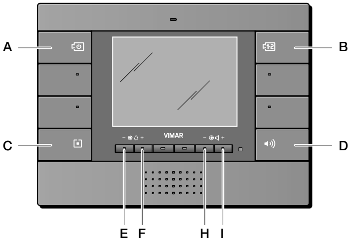
Figura 8 - Vista frontale monitor 01958.
