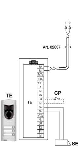
Figura 13 - Elettroserratura 12Vcc 200mA max
