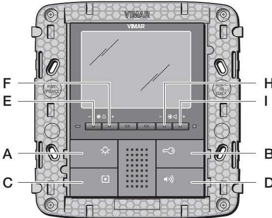
Figura 6 - Vista frontale monitor 20550.
