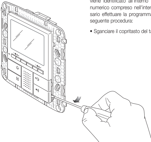
Figura 9 - Sgancio tasto
