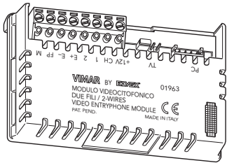
Figura 1 - Modulo videocitofonico 01963.
