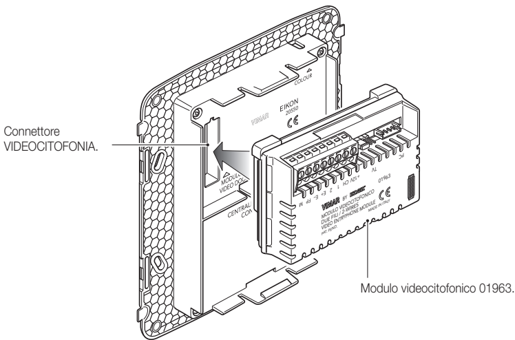
Figura 5 - Aggancio del modulo videocitofonico Due Fili.
