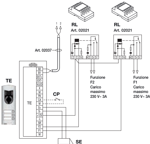
Figura 15 - Accensione luci scale con FUNZIONE F1/F2
