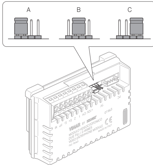
Figura 7 - Selettore di terminazione linea "TV"
