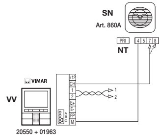
Figura 21 - Installazione con suoneria esterna Elvox
