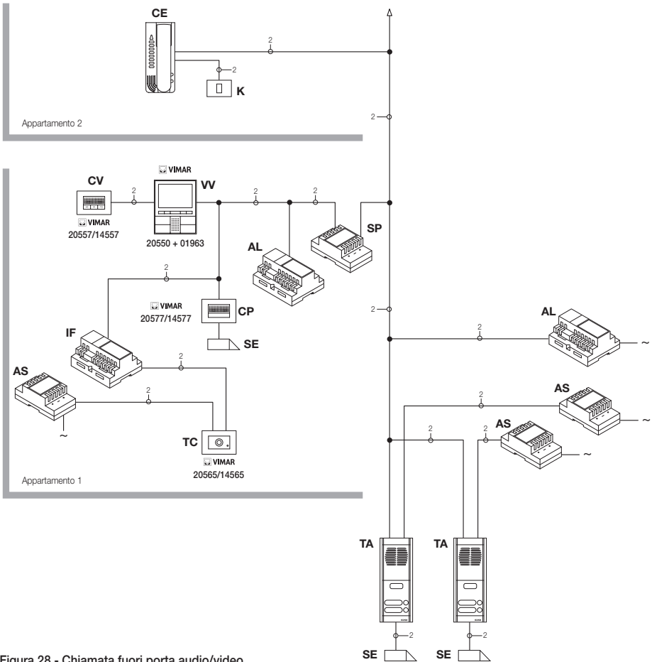
Figura 28 - Chiamata fuori porta audio/video
