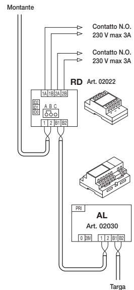
Figura 16 - Accensione luci scale con SERVIZIO AUX 1/2
