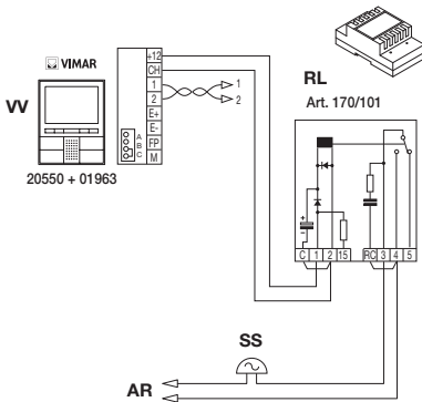
Figura 20 - Installazione suoneria esterna con relé
