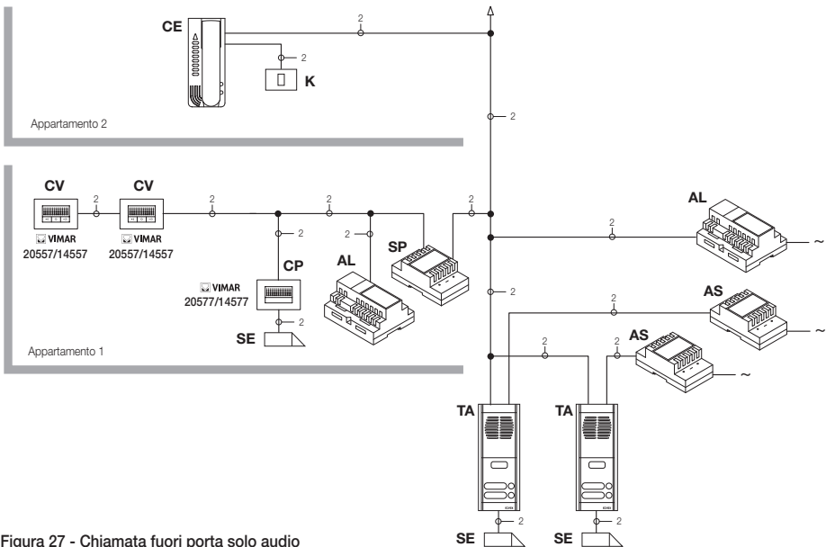
Figura 27 - Chiamata fuori porta solo audio
