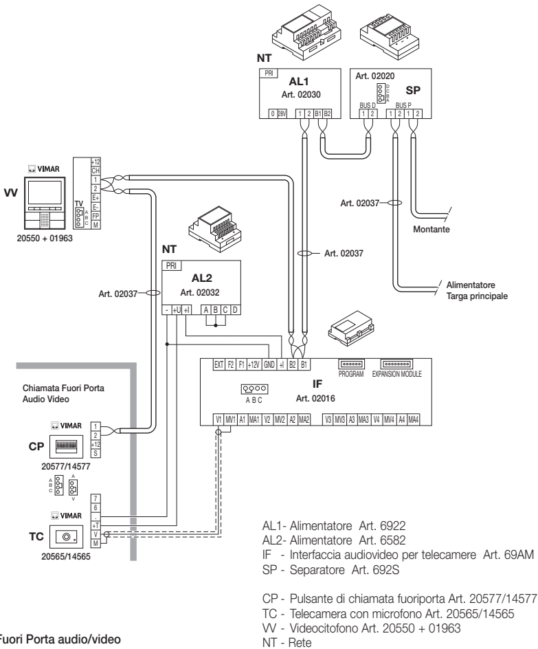
Figura 19 - Fuori Porta audio/video
