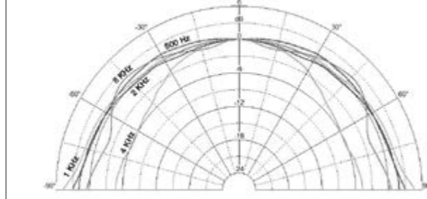
DIAGRAMMA POLARE - POLAR DIAGRAM - DIAGRAMME DES PÔLES DIAGRAMA POLAR - POLARDIAGRAMMA - ΠΟΛΙΚΟ ΔΙΑΓΡΑΜΜΑ
