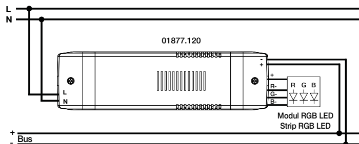
Abb. 1. Schaltbild des Netzteils 01877.120.
