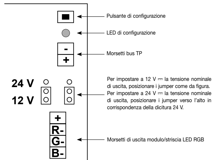
Fig. 2. Posizione dei jumper per selezionare la tensione di uscita a 12 V ~.
