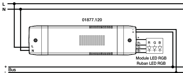
Fig. 1. Schéma des connexions d'alimentation 01877.120.
