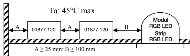
Abb. 3. Mindestabstände zwischen dem Netzteil 01877.120 und den Lampen und/oder Außenwänden.
