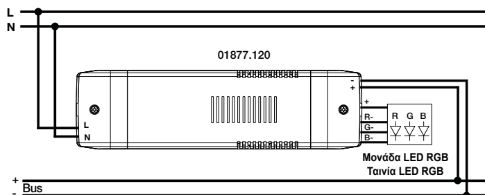
Εικ. 1. Διάγραμμα συνδέσεων τροφοδοτικού 01877.120.
