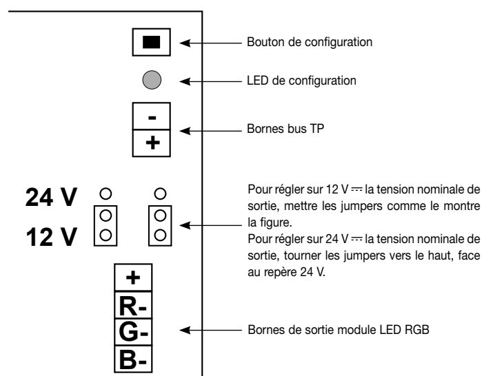
Fig. 2. Position des jumpers pour sélectionner la tension de sortie à 12 V ~.
