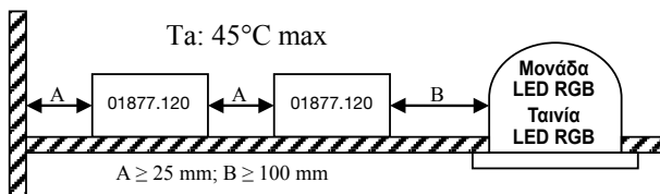
Εικ. 3. Ελάχιστες αποστάσεις μεταξύ τροφοδοτικού 01877.120 και λαμπτήρων ή/και εξωτερικών τοίχων.
