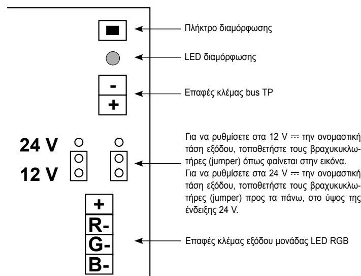
Εικ. 2. Θέση βραχυκυκλωτήρων (jumper) για επιλογή της τάσης εξόδου 12 V ~.
