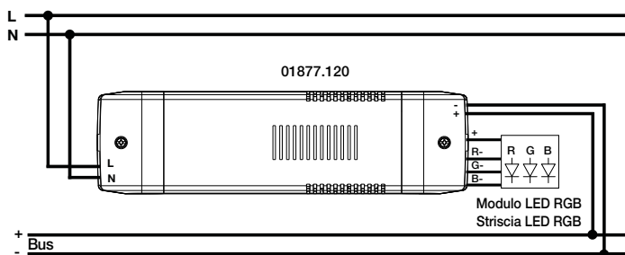
Fig. 1. Schema collegamenti alimentatore 01877.120
