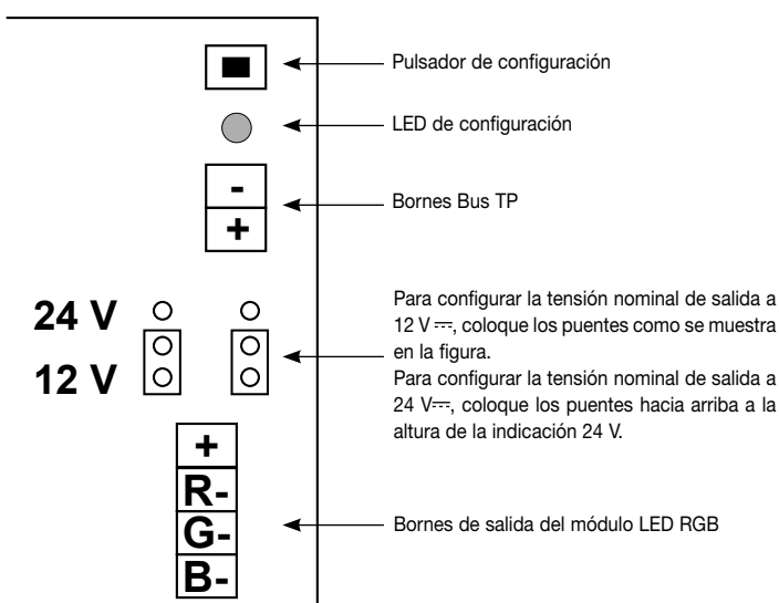
Fig. 2. Posición de los puentes para seleccionar la tensión de salida a 12 V ~.
