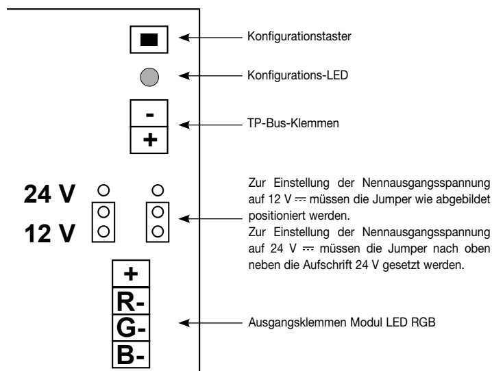
Abb. 2. Stellung der Jumper für die Wahl der Ausgangsspannung 12 V ~.
