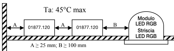
Fig. 3. Distanze minime tra l'alimentatore 01877.120 e le lampade e/o pareti esterne.
