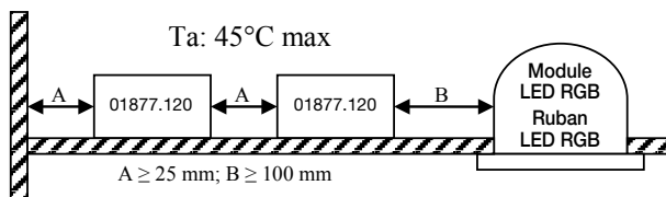
Fig. 3. Distances minimales entre l'alimentation 01877.120 et les luminaires et/ou les cloisons extérieures.
