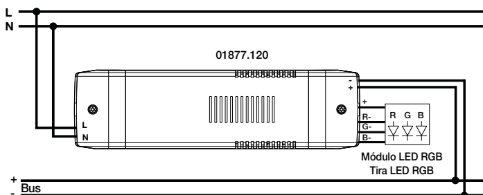
Fig. 1. Esquema de conexiones del alimentador 01877.120.
