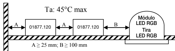
Fig. 3. Distancias mínimas entre el alimentador 01877.120 y las lámparas y/o paredes exteriores.
