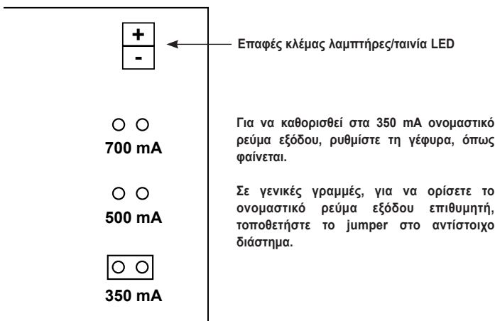
Εικ. 3 Θέση βραχυκυκλωτήρων για επιλογή του ρεύματος εξόδου 350 mA.
