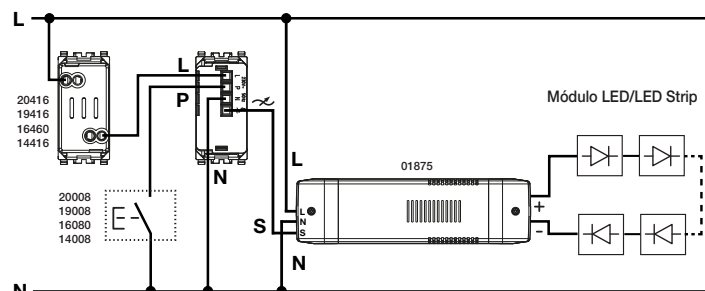
Fig. 1 Esquema de las conexiones del alimentador art. 01875 y el regulador master universal.
