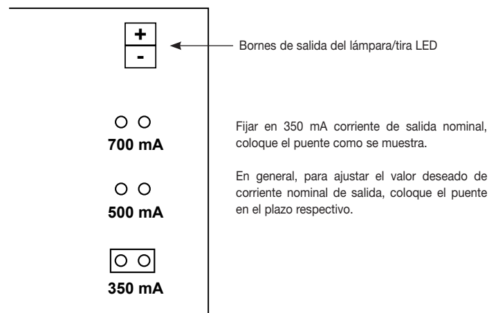
Fig. 3 Posición de los puentes para seleccionar la corriente de salida 350 mA.
