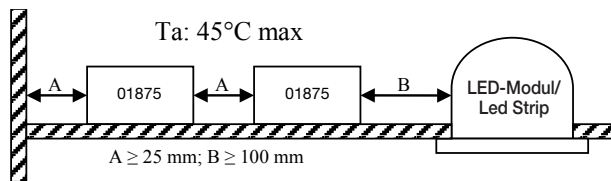
Abb. 4 Mindestabstände zwischen dem Netzteil 01875 und den Lichtern und/oder Außenwänden.
