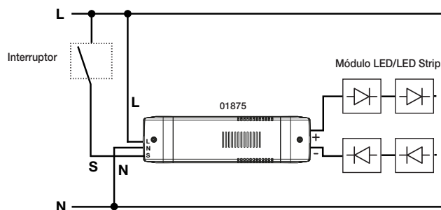
Fig. 2. Esquema de las conexiones del alimentador 01875 y el interruptor de encendido y apagado.
