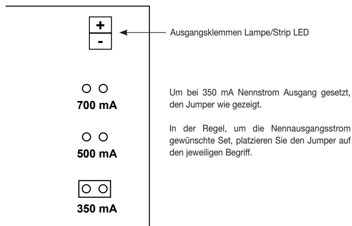
Abb. 3. Stellung der Jumper für die Wahl der Nennausgangsstromstärke 350 mA.
