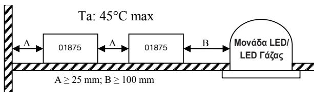
Εικ. 4. Ελάχιστες αποστάσεις μεταξύ του τροφοδοτικού 01875 και των φωτιστικών ή/και εξωτερικών τοίχων.
