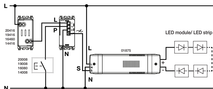
Abb.1. Schaltbild des Netzteils 01875 + Master-Universaldimmer.
