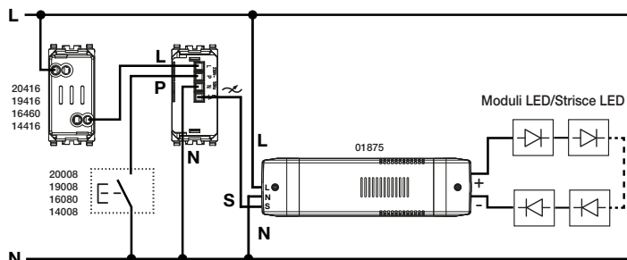
Fig. 1. Schema collegamenti alimentatore 01875 con regolatore master universale.
