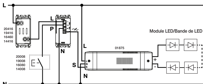
Fig. 1. Schéma de branchement de l'alimentation 01875 + variateur maître universel.
