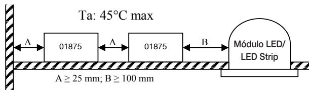
Fig. 4. Distancias mínimas entre el alimentador 01875 y las luminarias y/o paredes externas.
