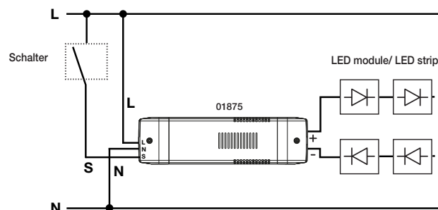
Abb. 2. Schaltbild des Netzteils 01875 + ON/OFF-Schalter.
