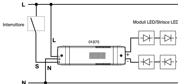
Fig. 2. Schema collegamenti alimentatore 01875 con interruttore ON/OFF.
