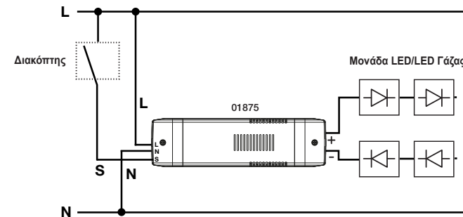
Εικ. 2 Διάγραμμα συνδέσεων τροφοδοτικού 01875 + διακόπτη ενεργοποίησης/απενεργοποίησης.
