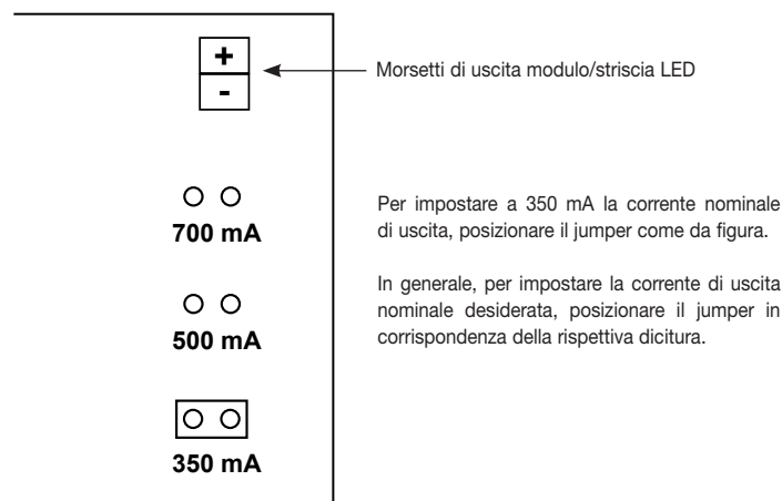
Fig. 3. Posizione del jumper per selezionare la corrente di uscita 350 mA.
