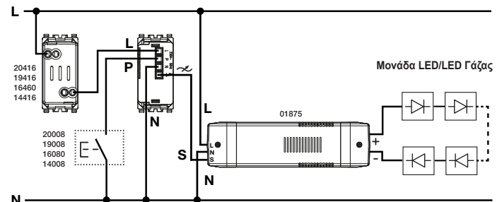
Εικ. 1 Διάγραμμα συνδέσεων τροφοδοτικού 01875 + ρυθμιστή master γενικού τύπου.
