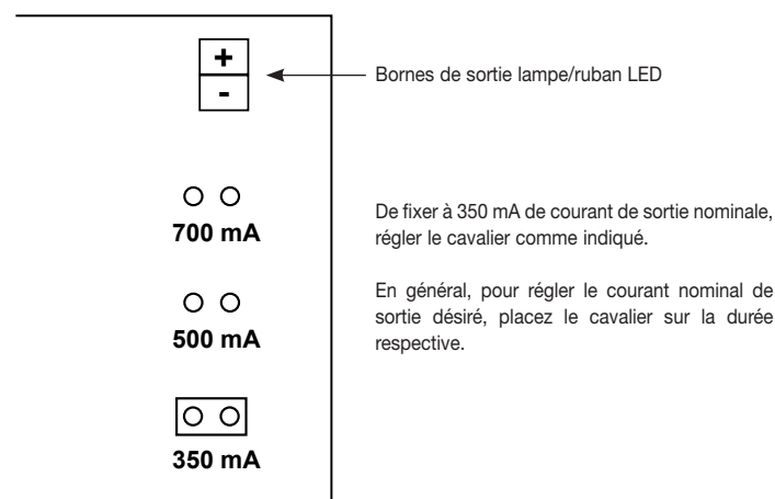
Fig. 3. Position des cavaliers pour sélection de la courant de sortie 350 mA.
