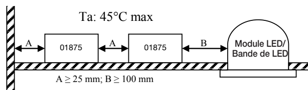
Fig. 4. Distances minimales entre l'alimentation 01875 et les luminaires et/ou les cloisons extérieures.
