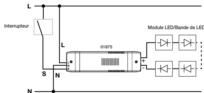
Fig. 2. 1 Schéma de branchement de l'alimentation 01875 + variateur maître universel.
