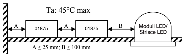
Fig. 4. Distanze minime tra l'alimentatore 01875 e le luminarie e/o pareti esterne.
