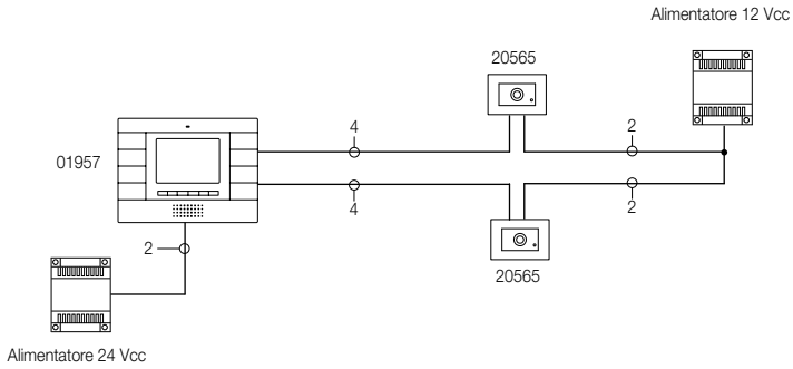
Figura 2 - Impianto TVCC con due ingressi audio/video
