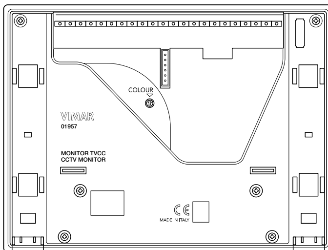
Figura 4 - Vista posteriore del monitor TVCC.
