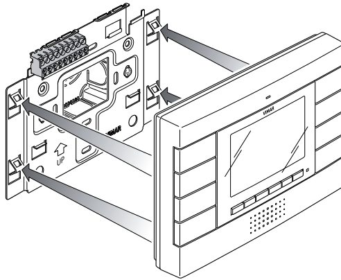
Figura 6 - Aggancio alla staffa
