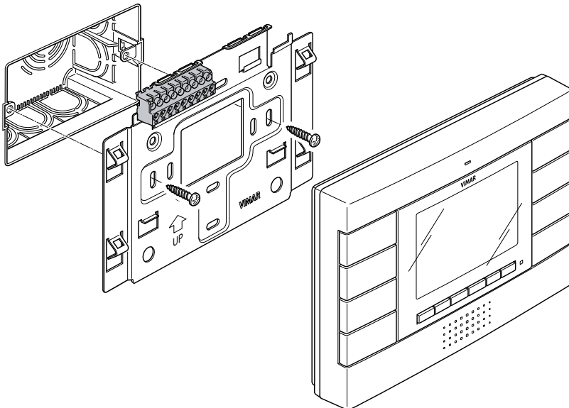
Figura 5 - Installazione della staffa sulla parete
