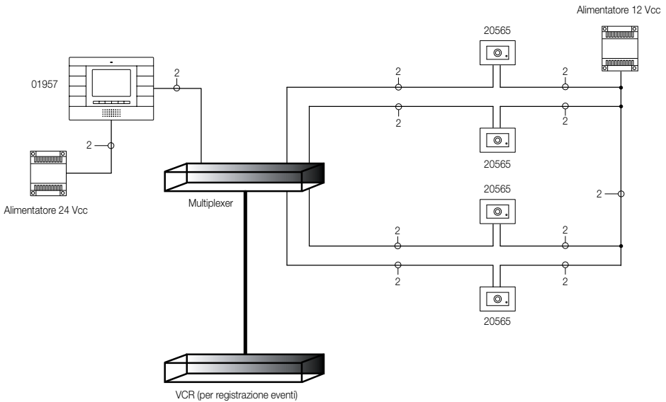
Figura 3 - Impianto TVCC con quattro ingressi video su multiplexer e VCR.
