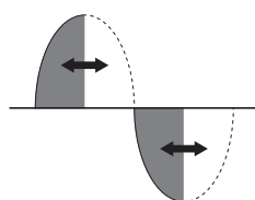
Dimmung mit Phasenabschnitt TE (Trailing Edge)
