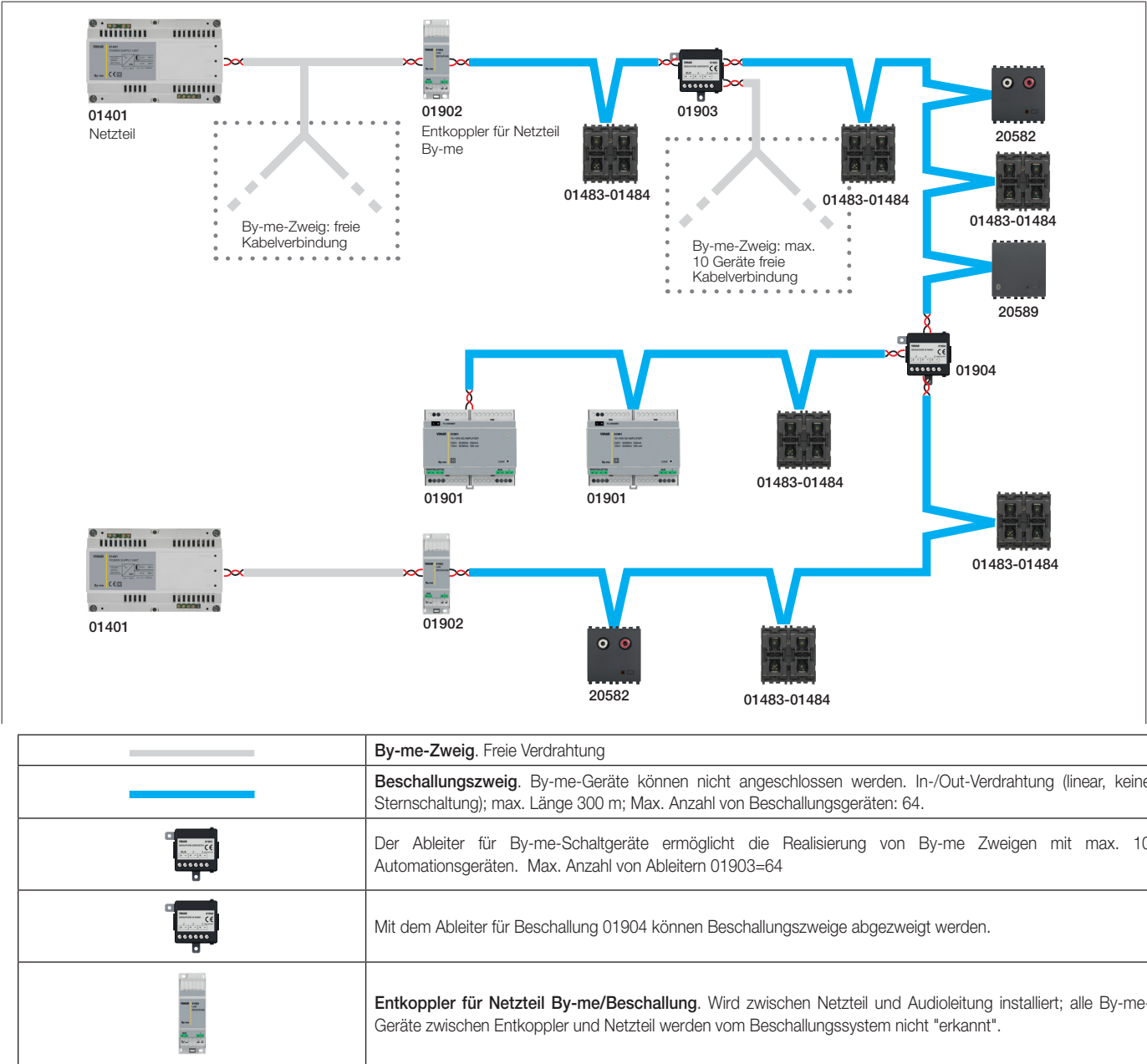
Beispiel 3: Beschallung und By-me-Automation auf dem gleichen Zweig
