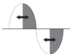
Dimmung mit Phasenanschnitt LE
