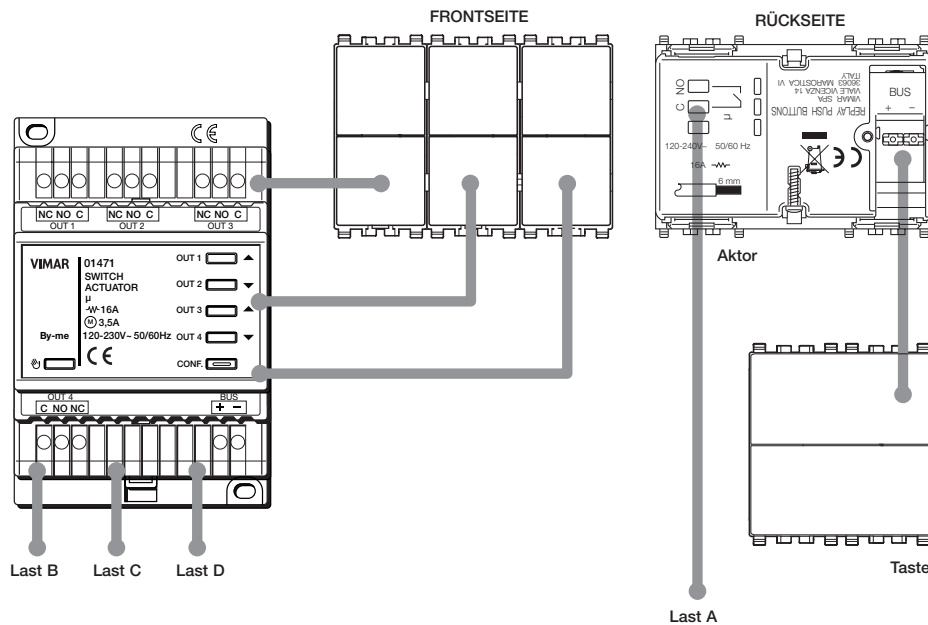
Schaltgerät mit sechs Tasten und Aktor Art. 30486-01486
