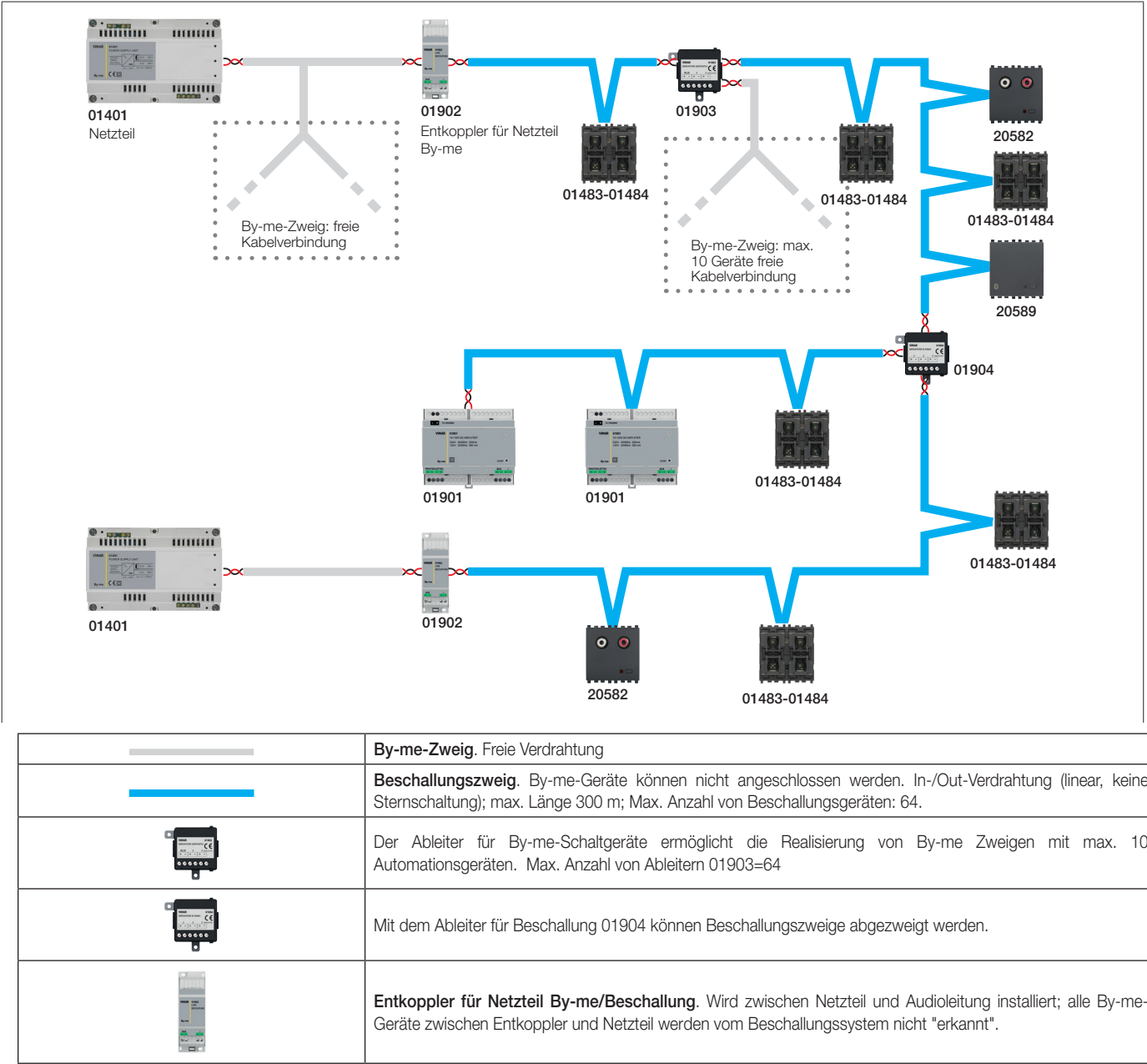
Beispiel 3: Beschallung und By-me-Automation auf dem gleichen Zweig
