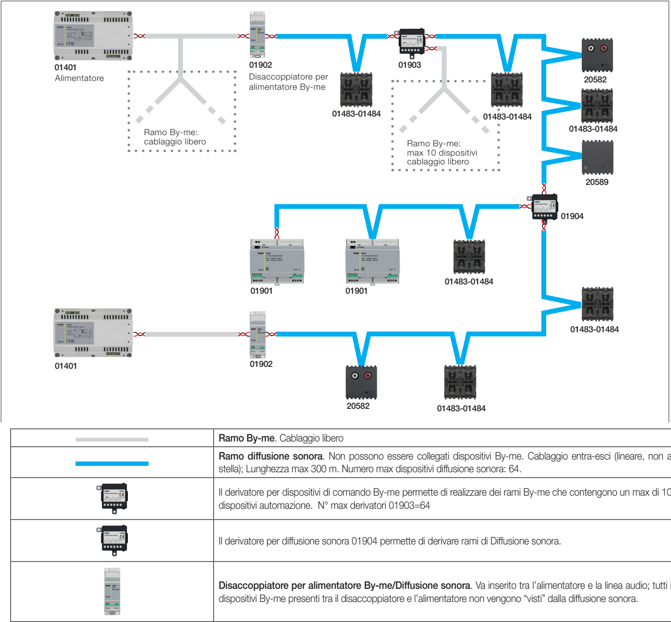
Esempio 3: diffusione sonora e automazione By-me sullo stesso ramo
