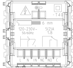
Vista posteriore
