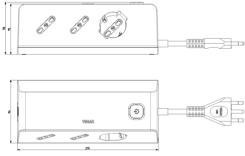
Vista ingombri
