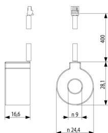
Vista ingombri
