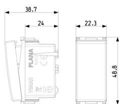
Vista ingombri
