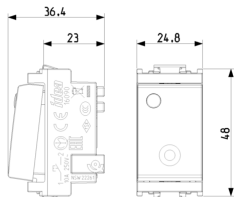
Vista ingombri
