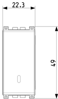
Vista ingombri
