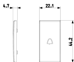
Vista ingombri
