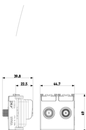
Vista ingombri
