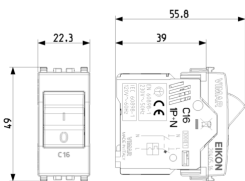
Vista ingombri
