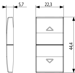
Vista ingombri
