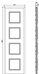
Vista ingombri
