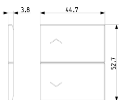
Vista ingombri
