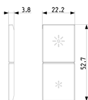
Vista ingombri
