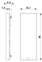
Vista ingombri
