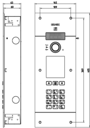
Vista ingombri
