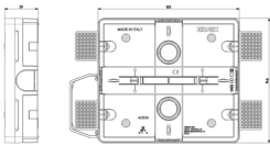
Vista ingombri
