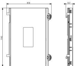
Vista ingombri
