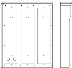
Vista ingombri
