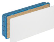
V70010 - Scatola derivazione incasso 515x201x80mm
