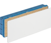
V70009 - Scatola derivazione incasso 479x154x70mm
